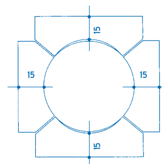
Oblò tondo Ø 44/54/60
